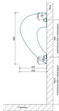
Technische Zeichnung für Urinaltrennwand „Imola“ aus HPL mit empfohlenen Höhenangaben (alle Angaben in mm)
