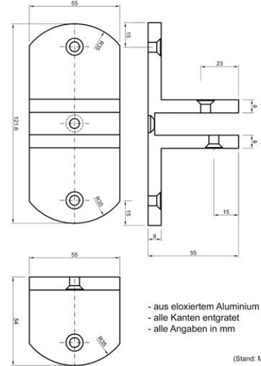
Technische Zeichnung des Plattenhalters für Urinaltrennwand „Imola“ aus HPL
