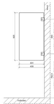
Technische Zeichnung für Urinaltrennwand aus HPL mit empfohlenen Höhenangaben (alle Angaben in mm)
