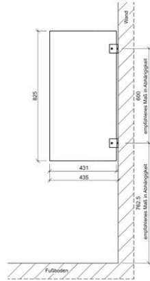
Technische Zeichnung für Urinaltrennwand aus Holzwerkstoff mit empfohlenen Höhenangaben (alle Angaben in mm)
