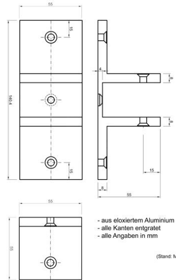
Technische Zeichnung des Plattenhalters für Urinaltrennwand aus Holzwerkstoff
