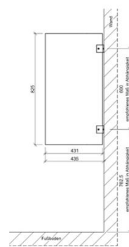
Technische Zeichnung für Urinaltrennwand aus Holzwerkstoff mit empfohlenen Höhenangaben (alle Angaben in mm)
