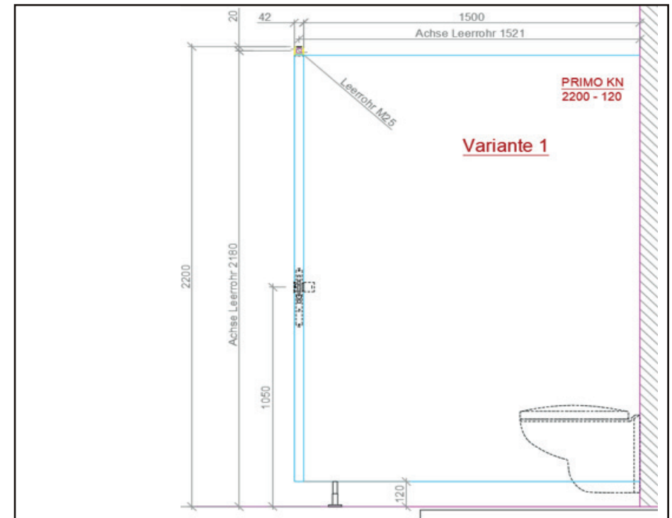
Toilettenanlage Innenraum, seitlich
