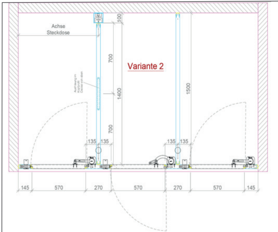
Einbündige Toilettenanlage, Türanschlag nach außen/innen
