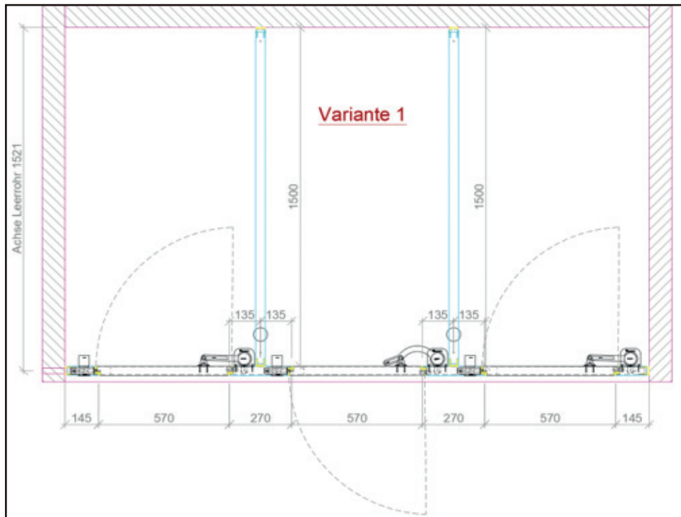
Einbündige Toilettenanlage, Türanschlag nach außen/innen
