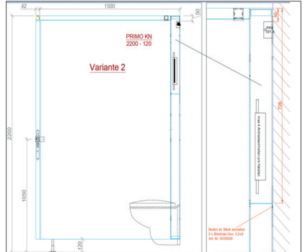
Toilettenanlage Innenraum, seitlich
